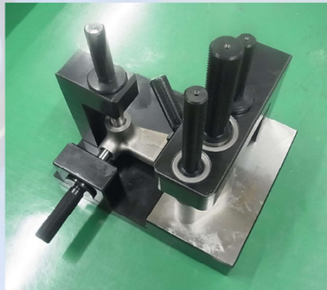
位置度測定ゲージ各種
